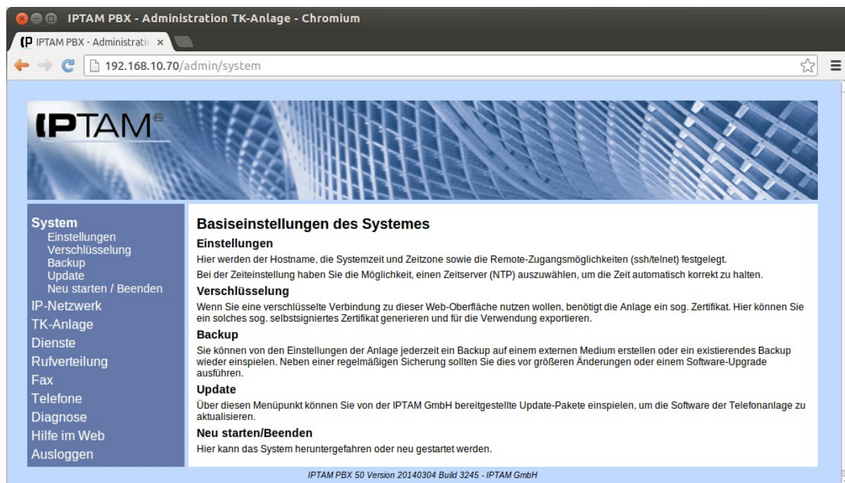
Abbildung 11.1.: Menü System
