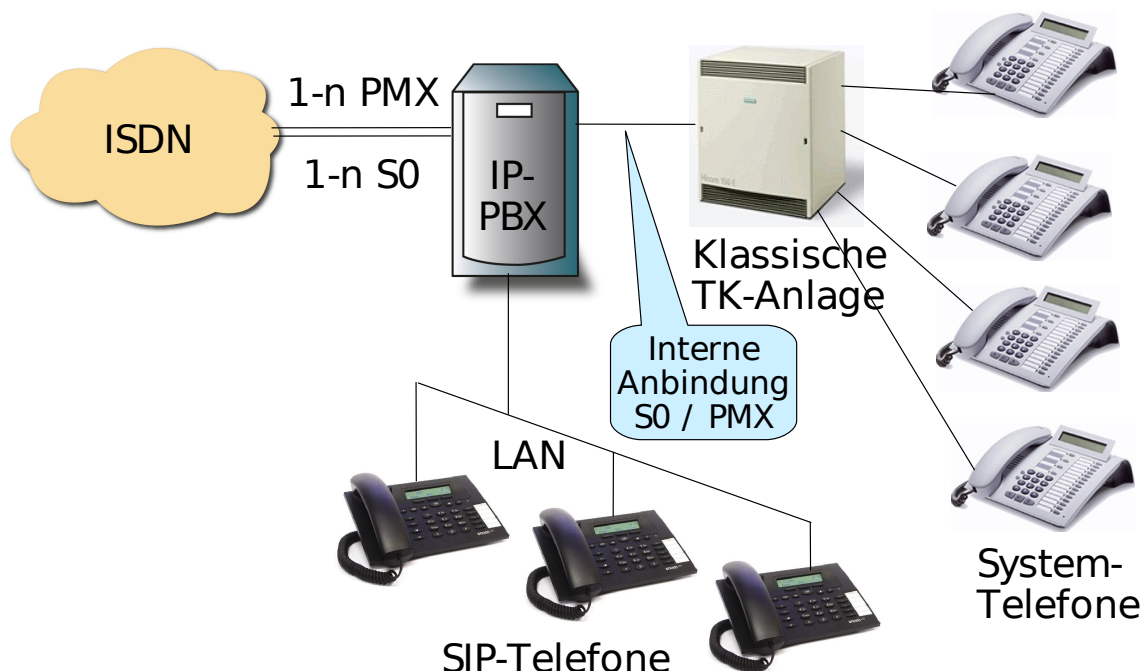
Abbildung 9.1: Anschluss bestehender ISDN TK-Anlagen an die IPTAM® PBX
