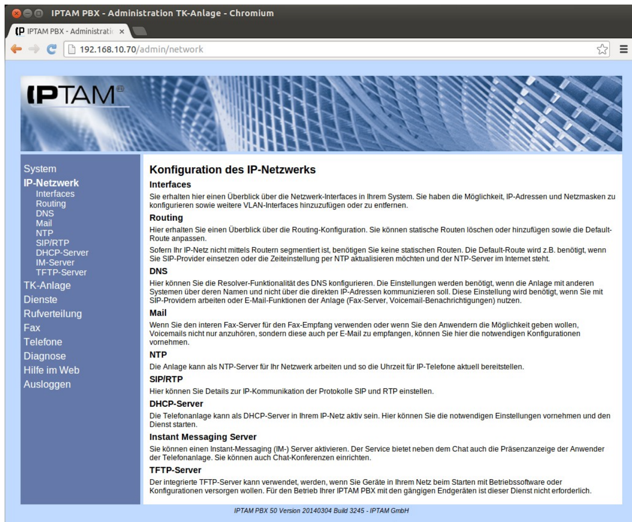
Abbildung 11.2.: Menü IP-Netzwerk
